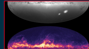
Diverse Ansichten des Himmels von Gaia
