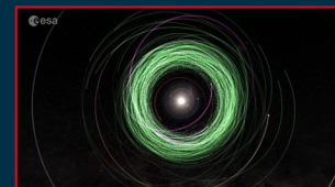
Entdeckung von Asteroiden durch Gaia
