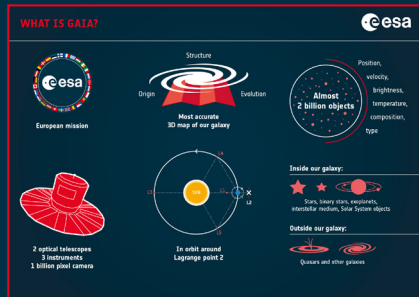
WAS IST GAIA?
