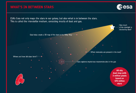
WAS ES ZWISCHEN DEN STERNEN GIBT
