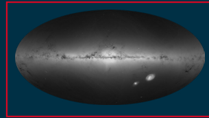
Dichte der Sterne
