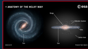
Anatomie der Milchstraße
