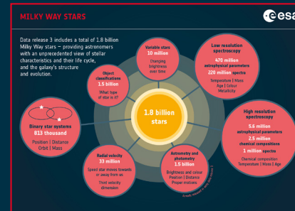
STERNE DER MILCHSTRASSE
