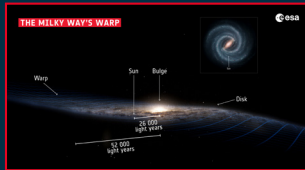
Verbiegung der Milchstraße
