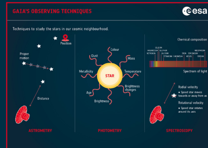
BEOBSACHTUNGSVERFAHREN VON GAIA
