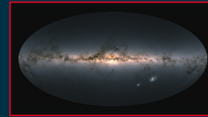
Farbe des Himmels
